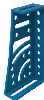
ESCUADRA DE SUJECIÓN PRO 275x500x175x100 16_N_016_PRO | 28_N_016_PRO
