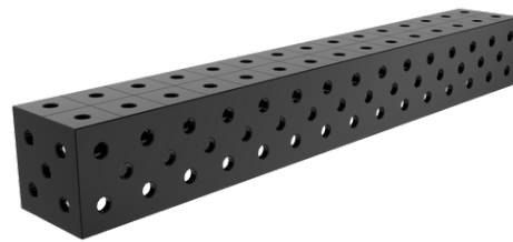
ПОДОВЖУВАЛЬНІ БЛОКИ ДЛЯ ЗВАРЮВАЛЬНИХ СТОЛІВ PLUS 1500X200X200
