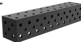
ΣΥΝΔΕΣΜΟΣ ΤΡΑΠΕΖΙΟΥ ΣΥΓΚΟΛΛΗΣΗΣ PRO 1000X200X200
