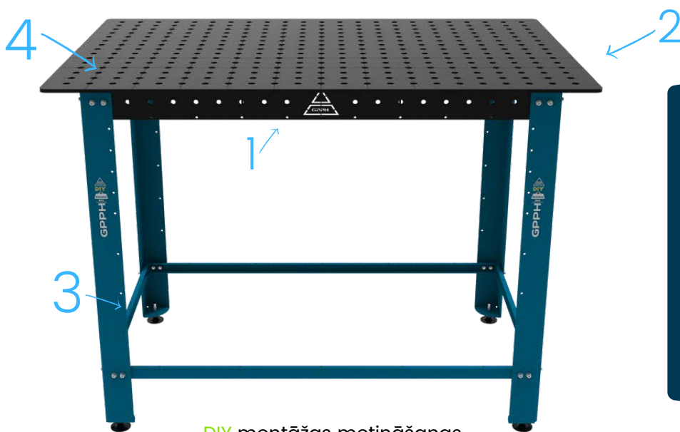
DIY montāžas metināšanas galds neto cena: 760 EUR
